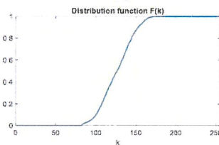
F1
